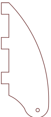
PER ALETTONI 2 PZ. PER ELEVATORE 1 PZ. SPESSORE 1,5 mm MULTISTRATO
