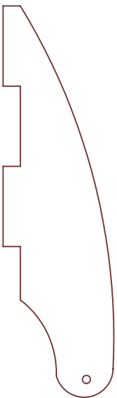
PER ALETTONI 2 PZ. PER ELEVATORE 1 PZ. SPESSORE 1,5 mm MULTISTRATO
