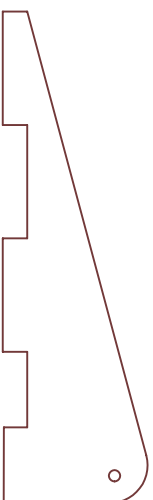
PER ALETTONI (INTERCONNESSIONE) 4 PZ. SPESSORE 1.5 mm MULTISTRATO
